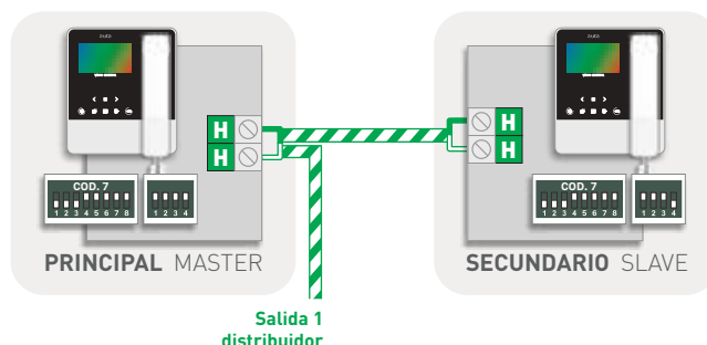
Manual de instalación SISTEMA 2H Installation manual 2W SYSTEM
