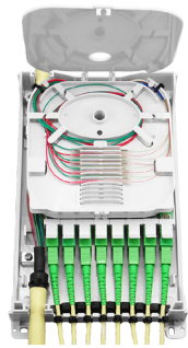
Fusión 8 cables 1FO 1 bandeja doble altura
