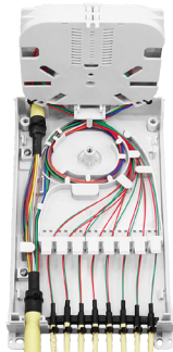
Salida fusiones desde 2 bandejas cable 2FO ICT2 a rosetas
