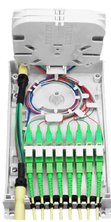
Salida inferior de pigtails 1FO con adaptadores
