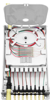
Fusión 4 cables 2FO ICT2 en 1 de las bandejas
