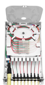
Fusión 8 cables 2FO ICT2 en 1 de las bandejas a doble altura
