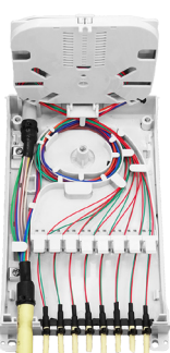
Salida fusiones desde 1 bandeja cable 2FO ICT2 a rosetas
