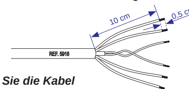
Dekoder-Bus Verdrahtung
