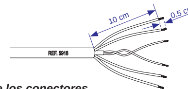
Cableado del BUS de DECODERS
